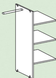
Vnitřní členění š x v x h (mm): 498x1662,5x534
