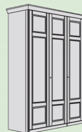
Šatní skříň 3 dveře Také provedení s1 a 3 zrcadly š x v x h (mm): 1605x2255x615
