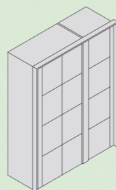
Šatní skříň, 3 dveře s římsou a lezénami š x v x h (mm): 1578x2201x627
